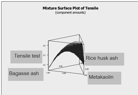
รูปที่ 7 ลักษณะพื้นผิวผลตอบส่วนผสมของการทดสอบความต้านทานแรงดึง
